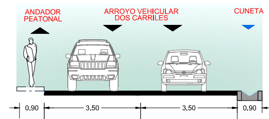
VIALIDAD COLECTORA (VC) 9.40m
