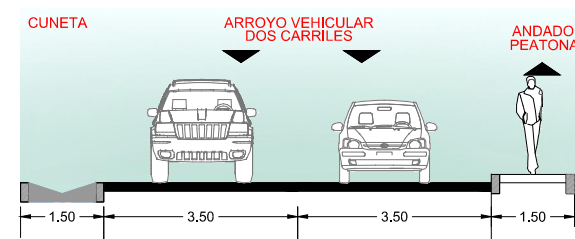
VIALIDAD SUBCOLECTORA (VSc) 10.00m
