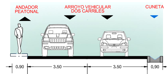
VIALIDAD LOCAL (VL) 9.40m
